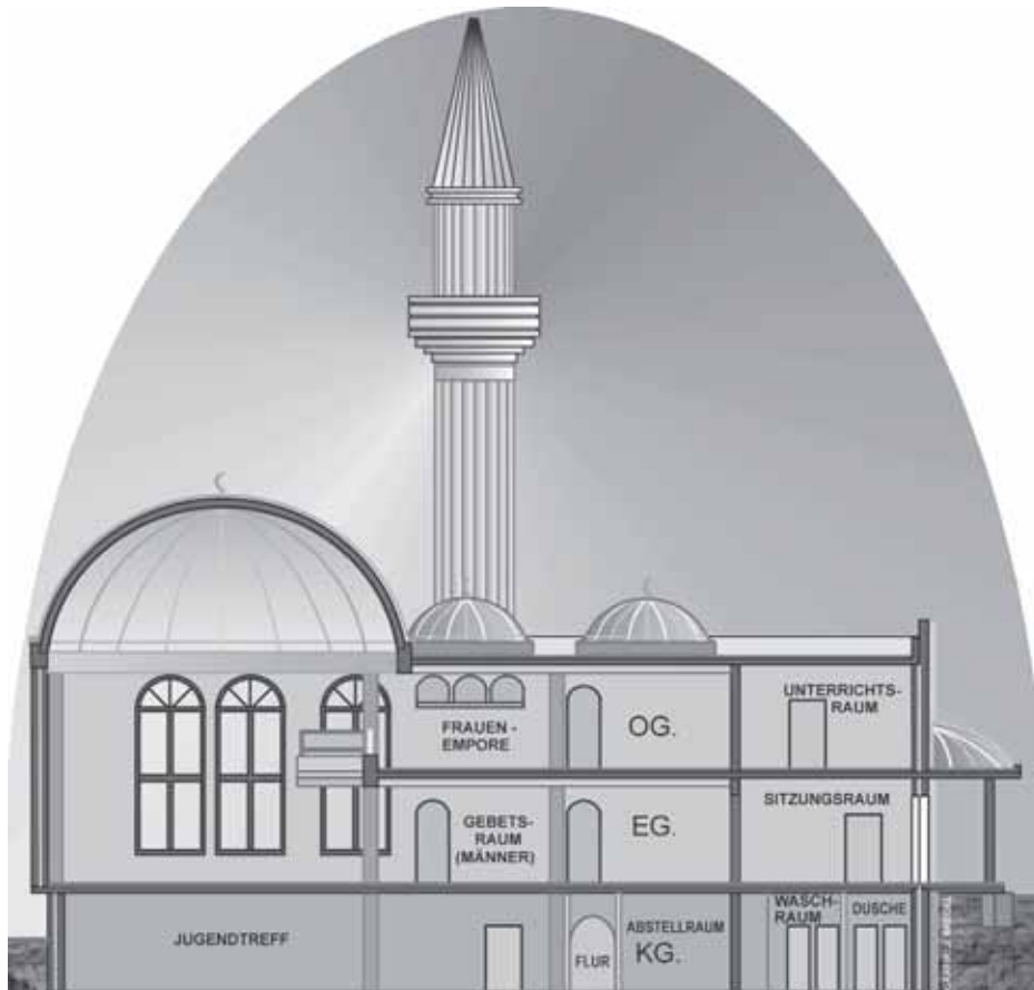
Abb. 2-3: Schnittzeichnung durch die Gladbecker Moschee Zeichnung: Jürgen Bregel, Bayreuth, nach einer Vorlage des Architekten Mustafa Erkal
